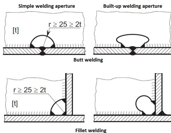
Fig. 12.16 Welding apertures
