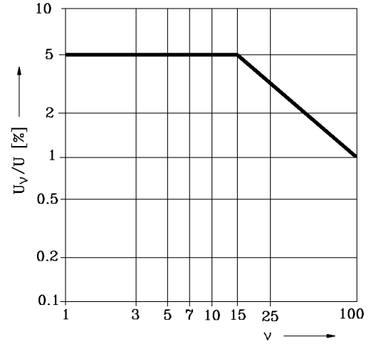
Şekil 1.1 Besleme gerilimindeki tekil harmonikler için sınır değerleri. U_v , v'inci gerilim harmoniğinin RMS değeridir
