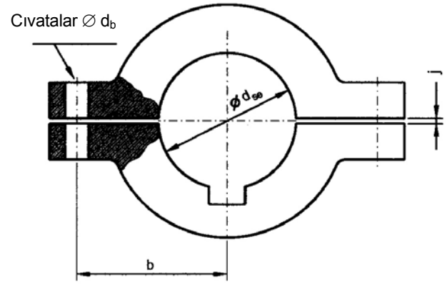
Şekil 7.7 Cıvatalı yekeler
