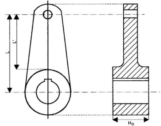
Şekil 7.6 Yeke kolu
