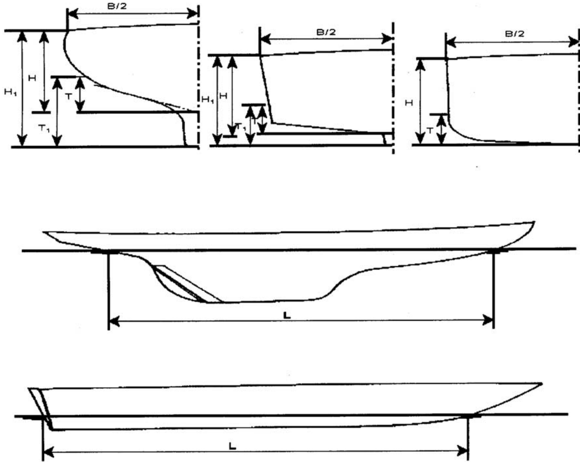
Şekil 2.1 Tekne boyutları
