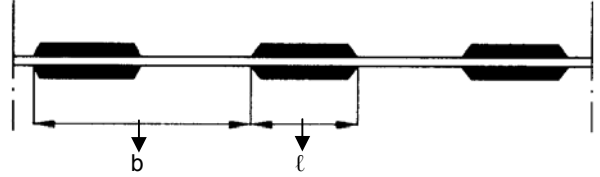
Şekil 5.1 Aralıklı zincir kaynağı
