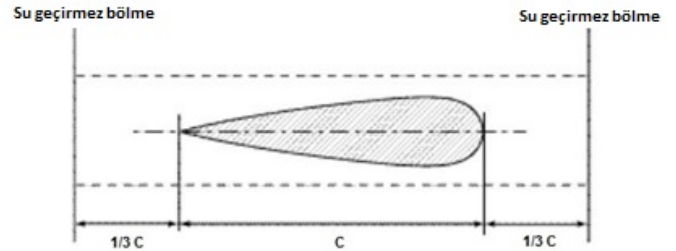
Şekil 2.5 Yalpa önleme kanatçığı konumlandırması
