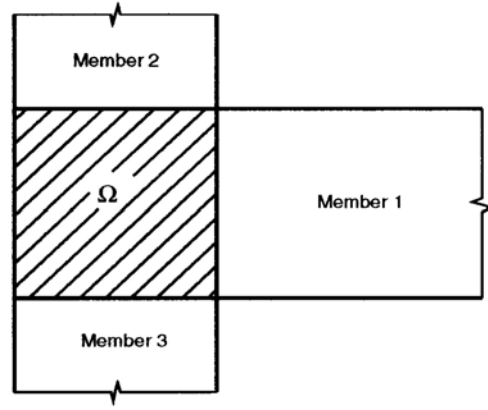
Şekil 5.18 Birincil taşıyıcı elemanların braketsiz uç bağlantıları
