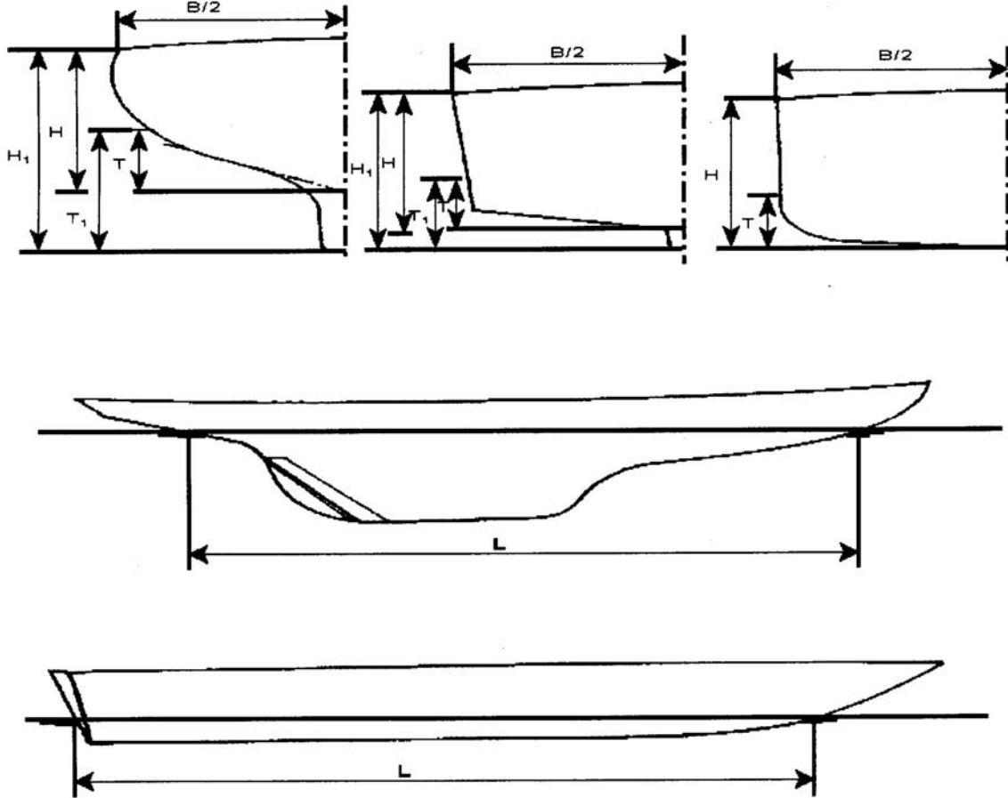
Şekil 2.1 Tekne boyutları
