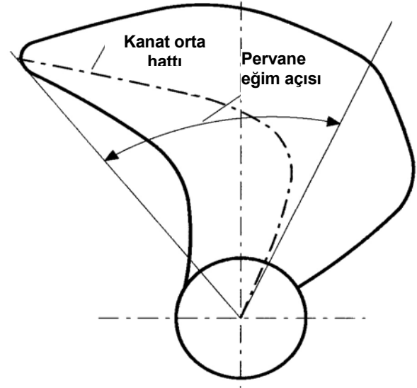
Şekil 7.4 Pervane çalıklığı (skew)
