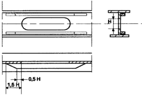
Şekil 5.20 Birincil taşıyıcı elemanlardaki büyük açıklıkların takviye edilmesi
