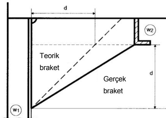
Şekil 6.6 Dik düzlemlerde yer alan stifnerlerin bağlantısı
