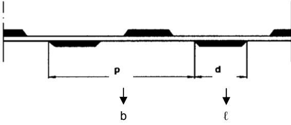
Şekil 5.3 Aralıklı zigzag kaynağı
