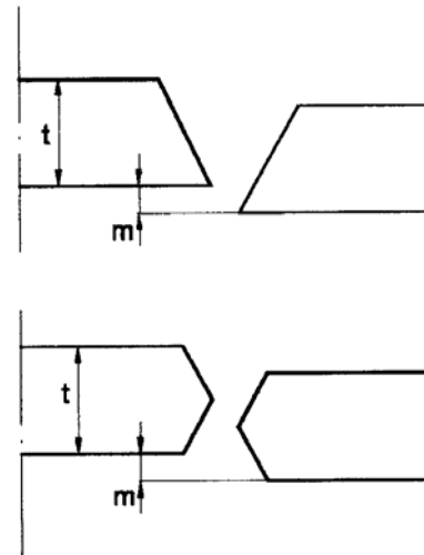
Şekil 5.11 Alın birleşiminde levha kaçıklığı
