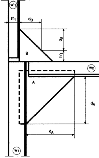
Şekil 5.28 Postaların kemerele bağlanması
