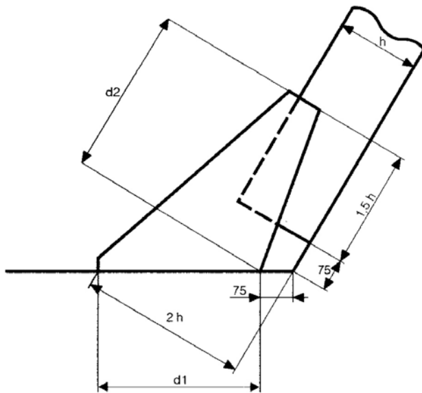
6.8 Postaların alt braketleri
