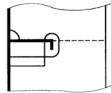
Şekil 5.13 Boğaz sacı olmaksızın normal takviye ile birincil takviye elemanının bağlantısı
