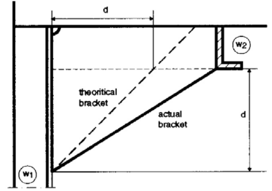
Şekil 5.27 Dik düzlemlerde yer alan stifnerlerin bağlantısı
