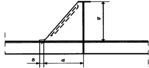
Şekil 5.22 Birincil taşıyıcı eleman: normal takviye bölgesindeki gövde takviyesi
