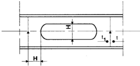
Şekil 5.21 Birincil taşıyıcı elemanlardaki büyük açıklıkların takviye edilmesi (insert levhası)
