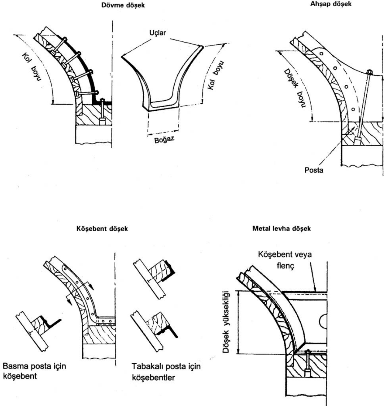
Şekil 3.6 Yelkenli Yatlar – Tipik Döşekler
