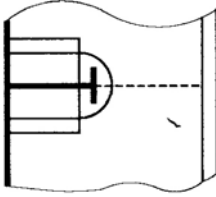
Şekil 5.16 Normal takviye ile birincil takviye elemanının iki büyük boğaz sacı ile bağlantısı
