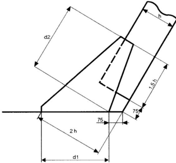
Şekil 5.29 Postaların alt braketleri
