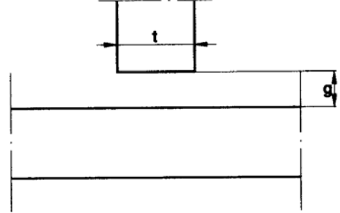
Şekil 5.10 İç köşe birleştirmesinde kök açıklığı
