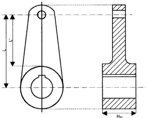
Şekil 7.6 Yeke kolu
