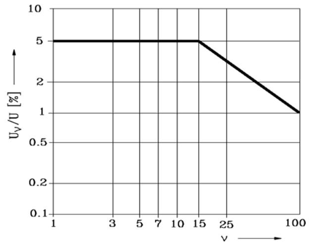
Şekil 1.2 Besleme gerilimi harmonikleri muafiyet sınırı U v , v inci sıranın gerilim harmoniklerinin RMS değeridir
