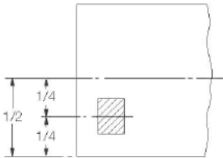
Şekil 3.13 Levhalar ve yassı elemanlar
