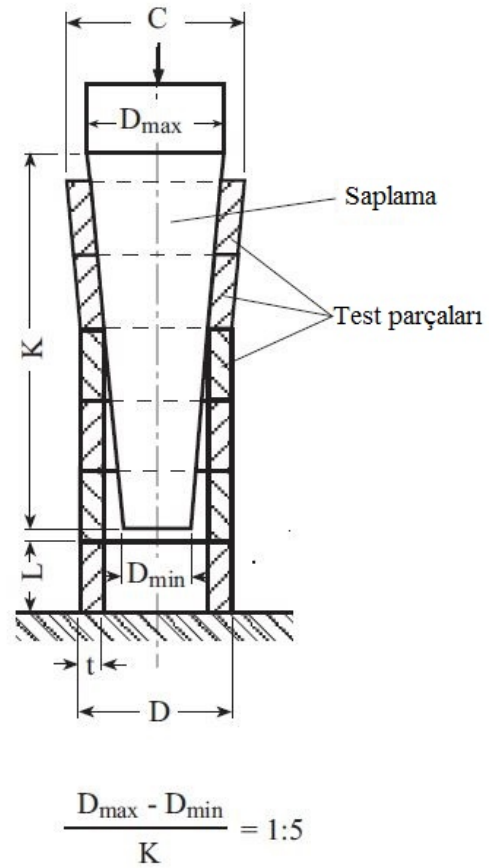
Şekil 2.12 Halka genişletme testi
