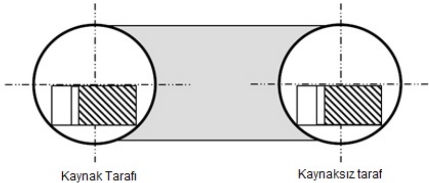
Şekil 10.6 CTOD test numunelerinin yerleri
