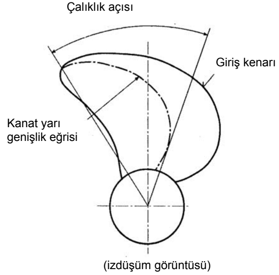
Şekil 11.2 Kanat çalıklık açısının tanımı
