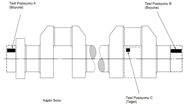
Şekil 5.4 Krankşaftta test numunelerinin yeri
