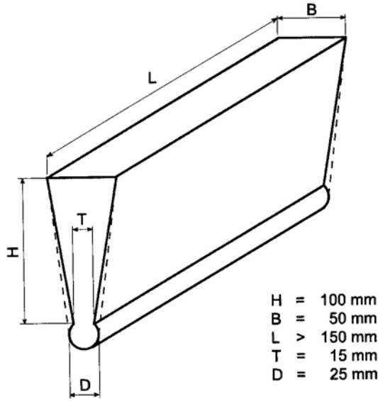
Şekil 11.1 Test parçası dökümü
