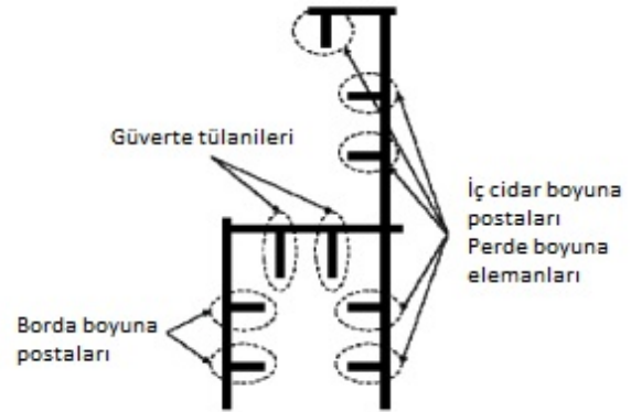
Şekil 3.14 Üst flenç boyuna yapısal elemanları
