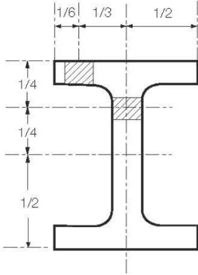
Şekil 3.6 H-Profil
