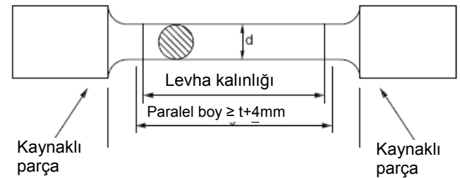
Şekil 3.11 Kaynaklı test numunesi
