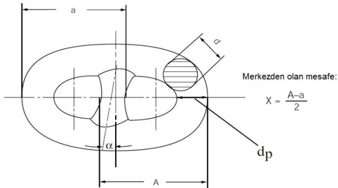
Şekil 10.3 Üretim toleransları
