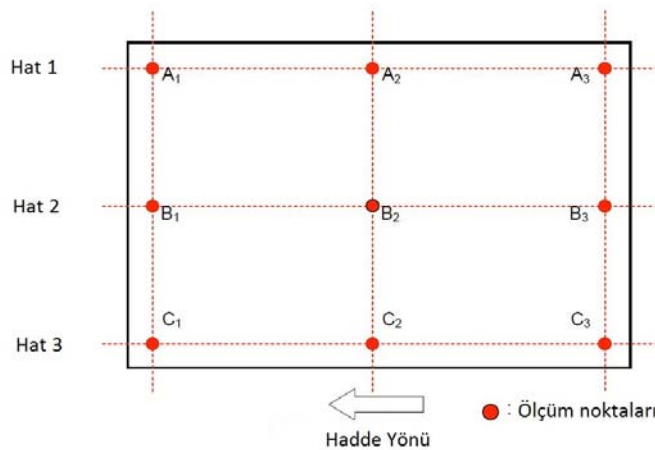
Şekil 3.1a Orjinal çelik levhalar için kalınlık ölçüm noktalarının yerleri
