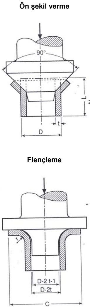
Şekil 2.11 Flençleme testi
