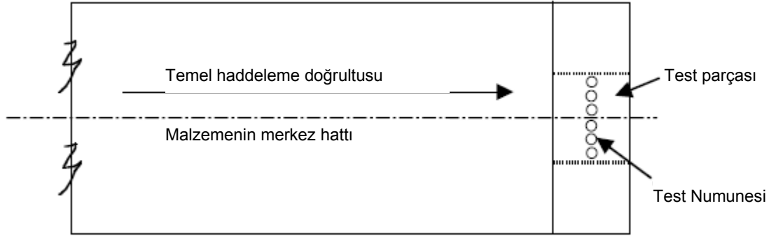
Şekil 3.9 Levha ve geniş lama parça alma yerleri
