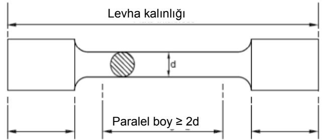
Şekil 3.10 Normal test numunesi
