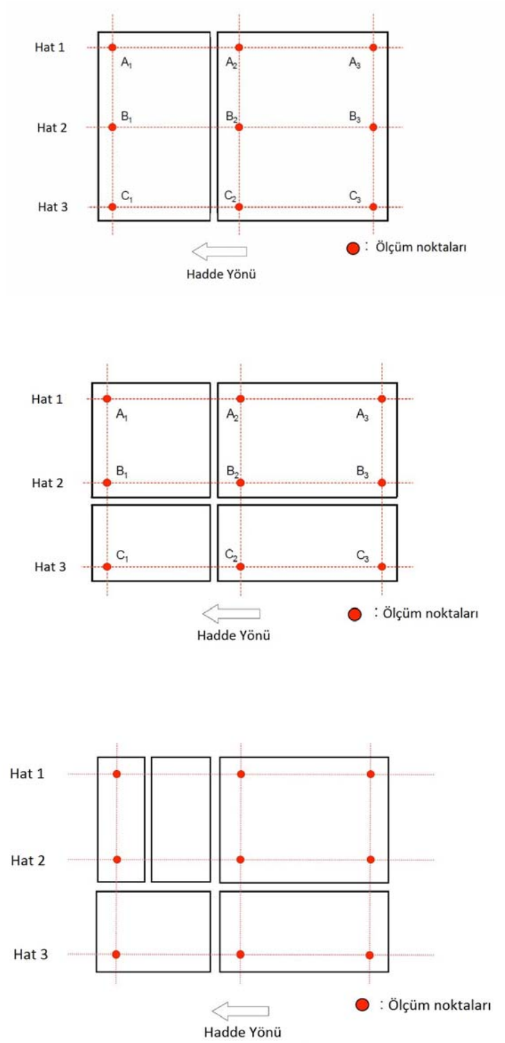
Şekil 3.1b Kesilmiş çelik ürünler için kalınlık ölçüm noktalarının yerleri
