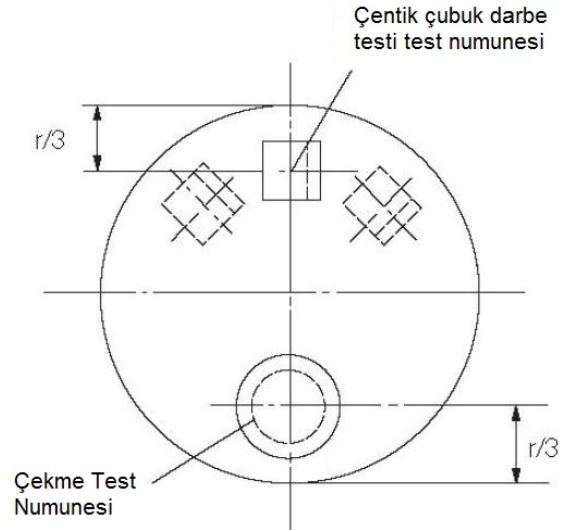
Şekil 10.7 Çelik çubuklar, dövme ve dökümlerden örnek alınması
