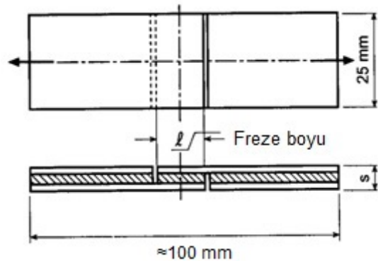
Şekil 12.2 3 katlı kontrplak levhalarda boyuna test parçaları
