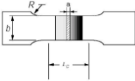
Şekil 2.6 Alın kaynağı çekme testi test numunesi
