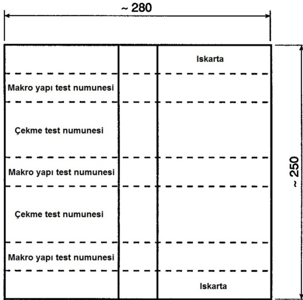
Şekil 11.A.1 Test parçası
