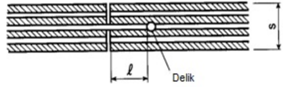
Şekil 12.7 7 katlı kontrplak levhalarda enine test parçaları
