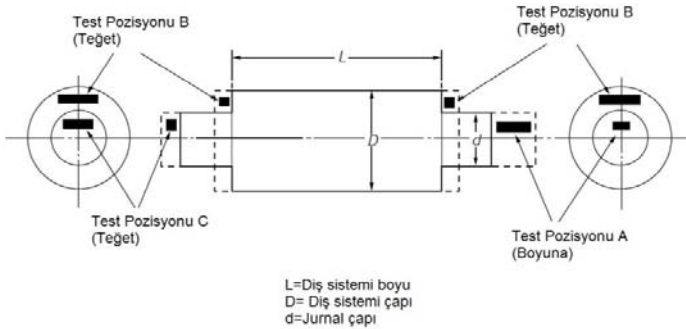
Şekil 5.5 Pinyon
