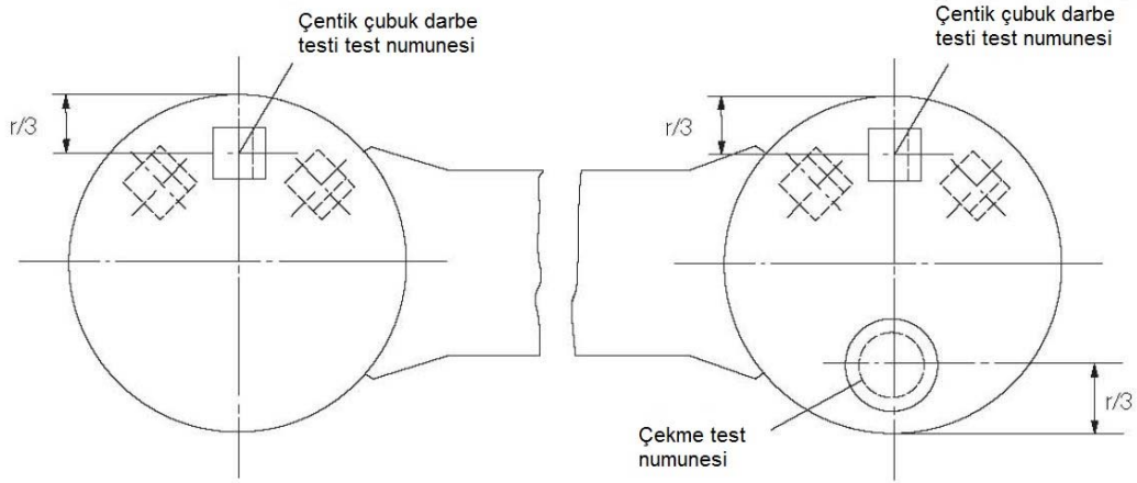
Şekil 10.8 Zincir baklası test parçasının alınması
