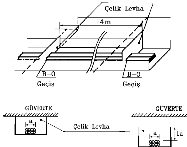
Şekil 12.2 Yarım kapalı dikey kanallar
