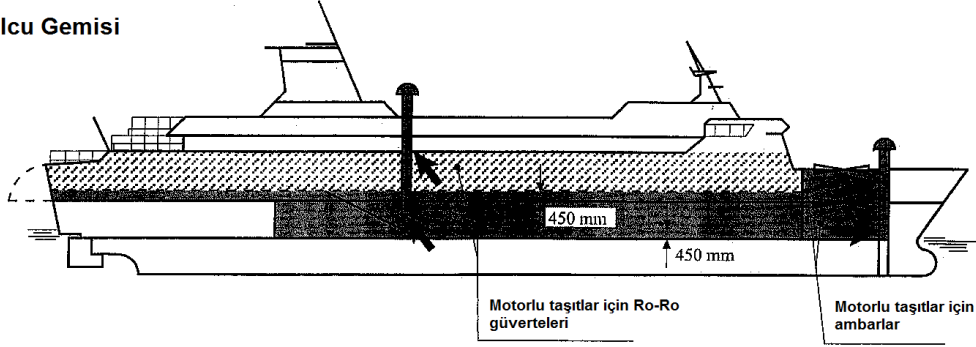
Ro-Ro Kargo Gemisi
