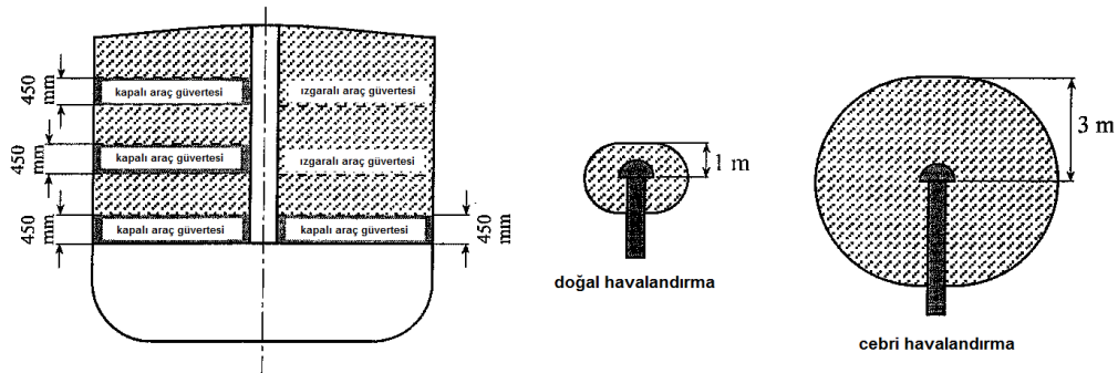
Motorlu taşıtlar için Ro-Ro güverteleri
