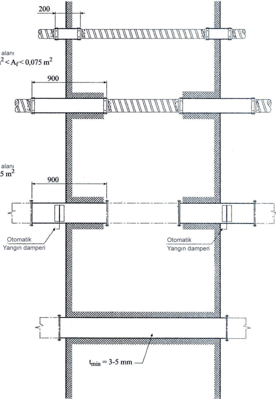
Şekil A.1 "A" sınıfı perdeden kanal geçişi ayrıntıları
